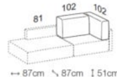
Cod. (&lt;-) E-ZCSA7S - E-ZCSA7D (-&gt;)
